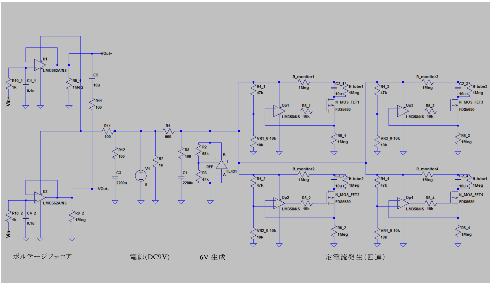
微小定電流装置基本回路図(4出力, ボルテージフォロア付き)
